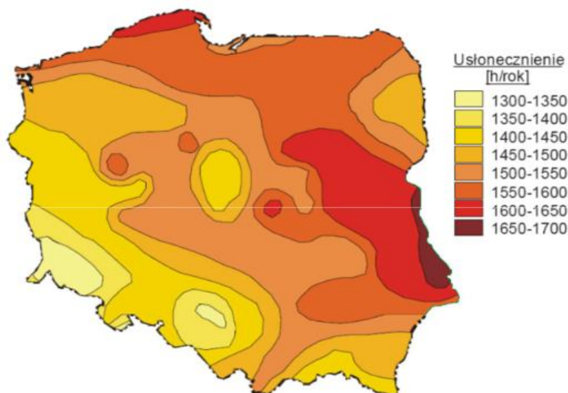
Ryc. 19. Średnie roczne sumy uśłonecznienia w Polsce
